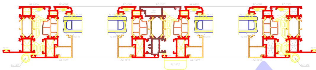
Fig. 2B: sezione orizzontale del campione pervenuto e sottoposto a prova (dimensioni nominali dichiarate, espresse in mm)
