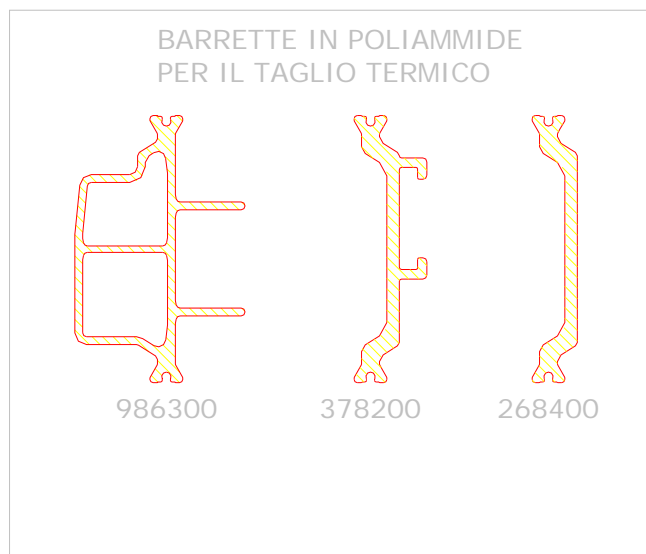
Fig. 4B: Dettagli del taglio termico del campione pervenuto e sottoposto a prova
