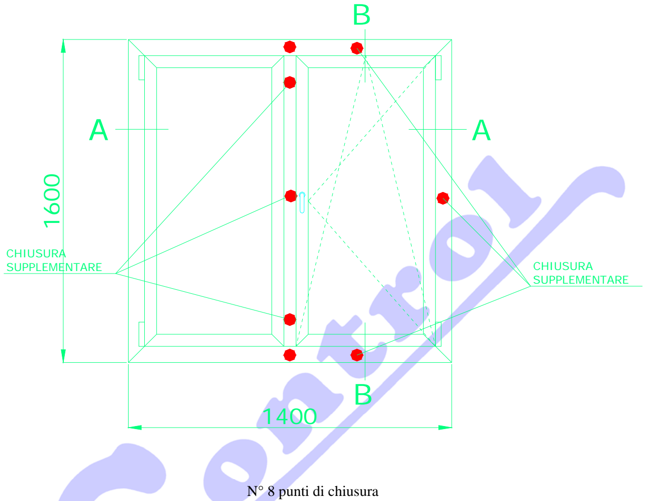
Fig.1b: punti di chiusura del prospetto del campione pervenuto e sottoposto a prova
