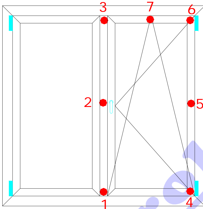
Fig. 5: Assetto sperimentale prova di resistenza al carico del vento: schema di posizionamento dei trasduttori (vista interna) 1-2-3 Montante A 4-5-6 Montante B 3-7-6 Traverso C
